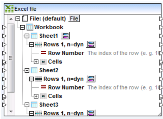
Excel-Standardkomponente
