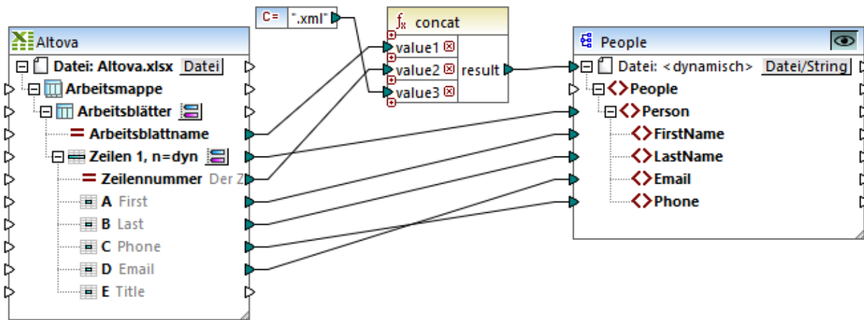
ConvertExcelRows.mfd (Teil 2)
