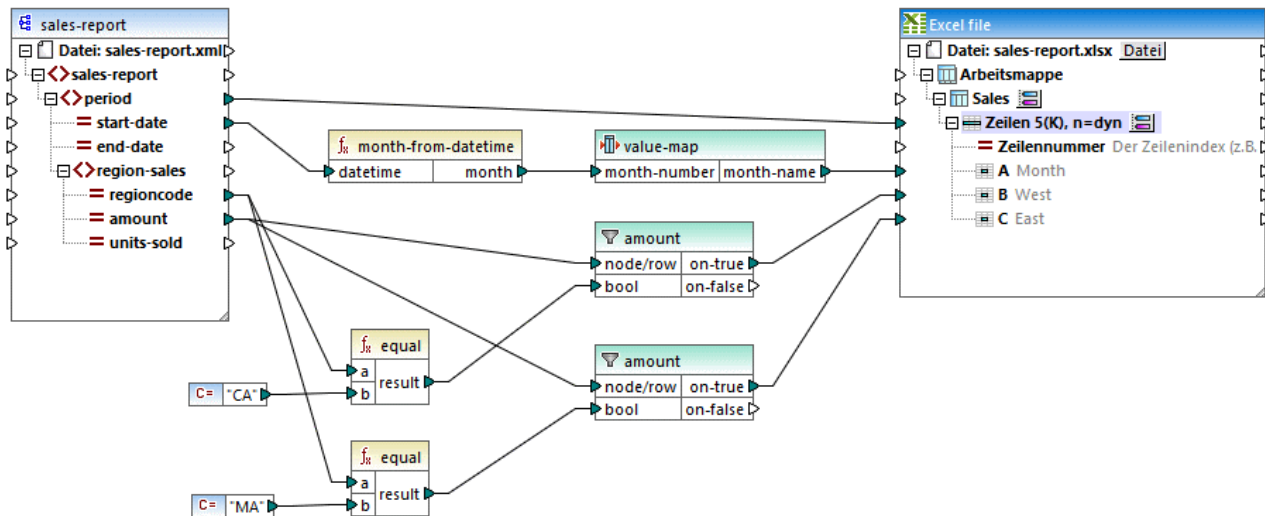
Sales_to_Excel.mfd
