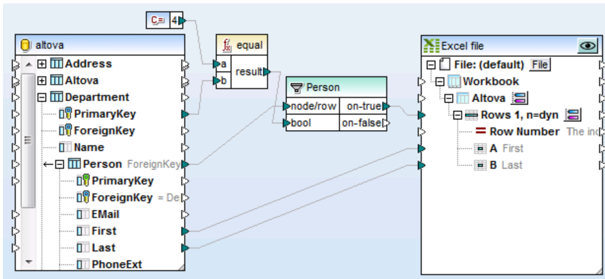
Excel-mapping.mfd (Beispiel 3)
