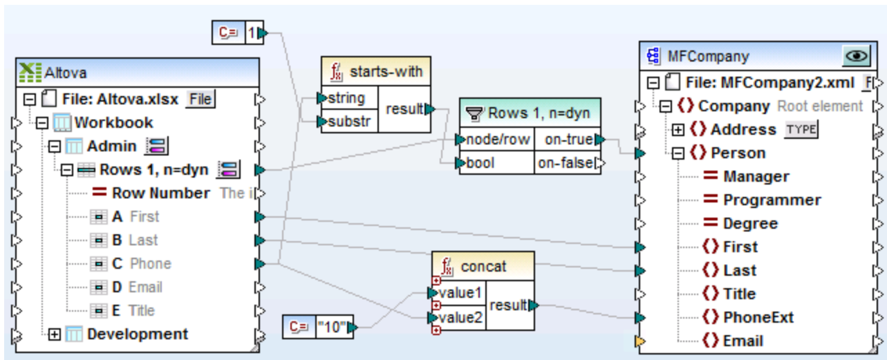
Excel-mapping.mfd (Beispiel 2)
