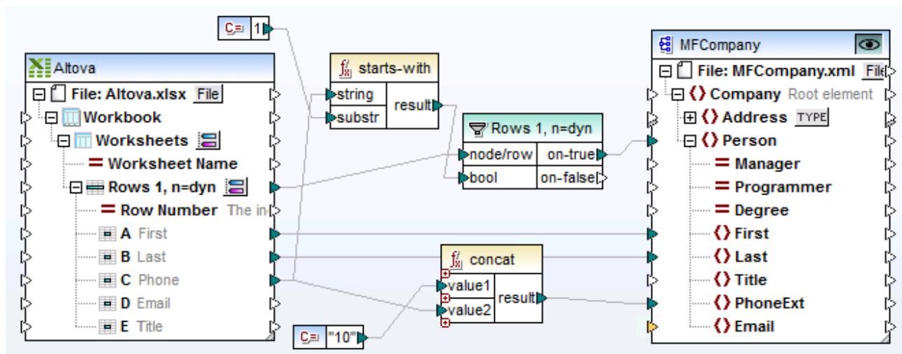
Excel-mapping.mfd (Beispiel 1)
