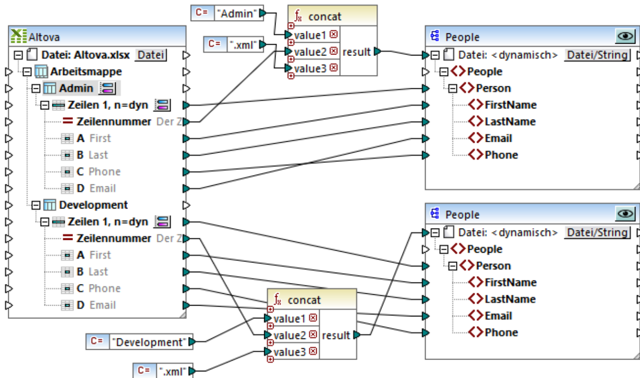
ConvertExcelRows.mfd (Teil 1)
