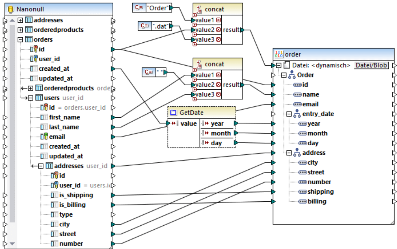
GenerateOrders.mfd
